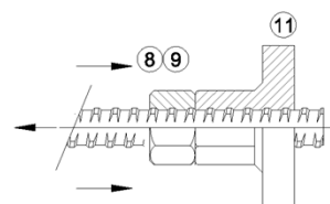
Bild 3 Ø12 - 50
