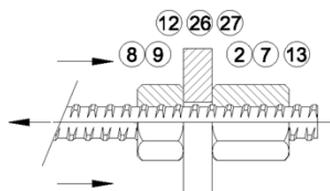
Bild 1 Ø12 - 50
