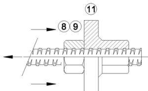
Bild 2 Ø12 - 50
