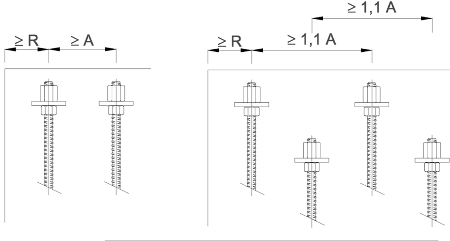
versetzte Verankerung
