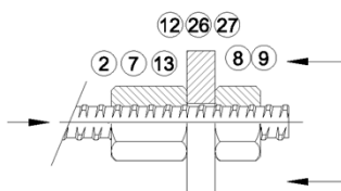
Bild 4 Ø12 - 50
