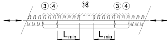
Bild 7 Muffenstoß - Sechskantmuffe, lang Ø12 - 50
