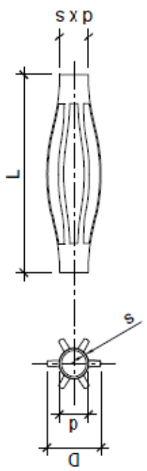
Detail 1 Abstandhalter
