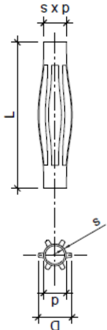
Detail 1 Abstandhalter
