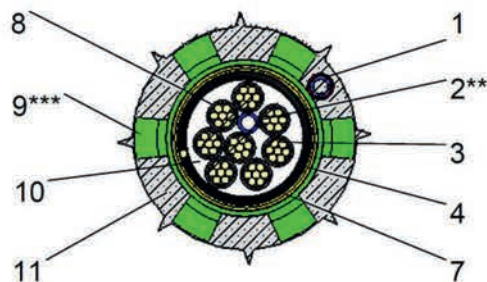
Schnitt B-B (innerhalb L_{tb} )
