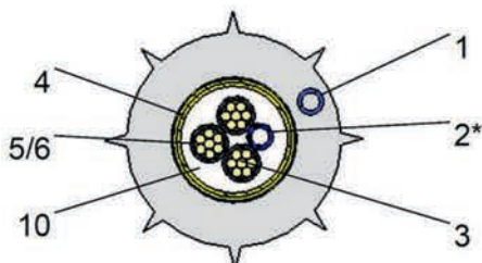
Schnitt A-A (innerhalb L_{tf} )
