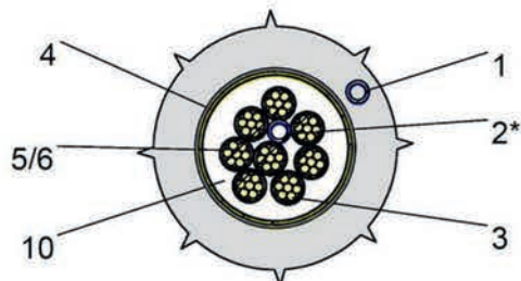
Schnitt A-A (innerhalb L_{tr} )
