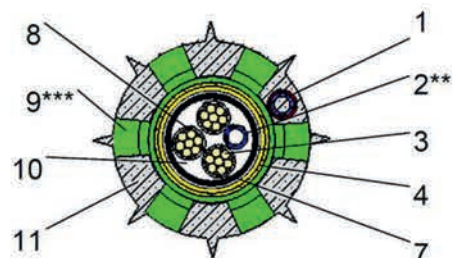
Schnitt B-B (innerhalb L_{tb} )
